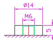
M6 Bolt B3 Terminal
